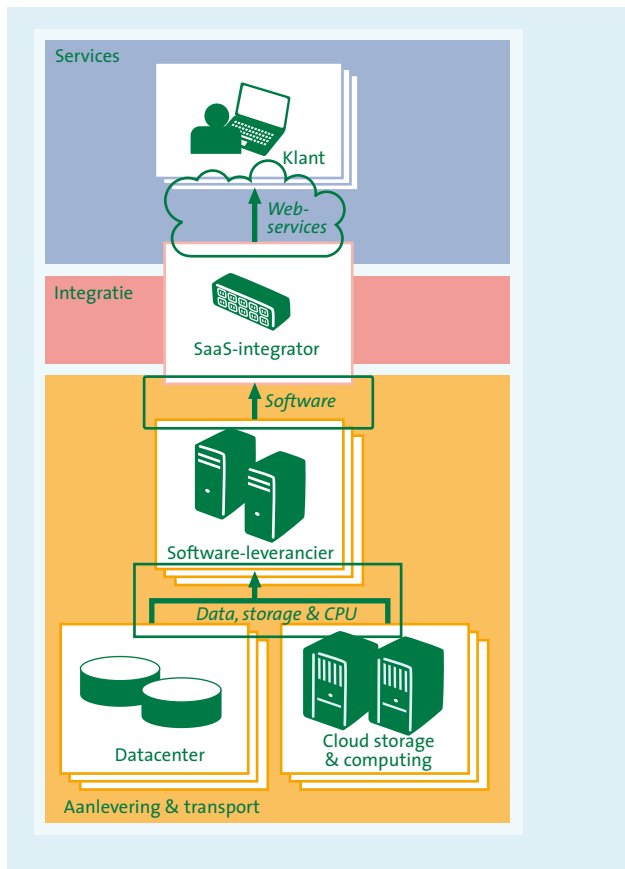
Figuur 4. 'Multi-instance'-architectuur.
