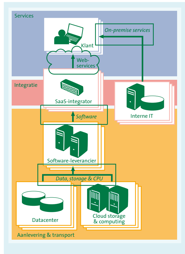
Figuur 5. 'Multi-integration'-architectuur.
