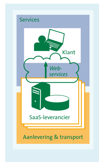
Figuur 3. 'Multi-vendor'-architectuur.
