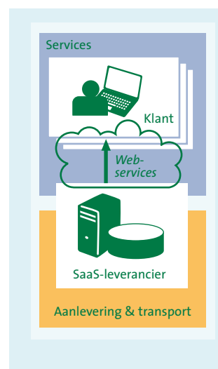
Figuur 2. 'Multi-tenant'-architectuur.
